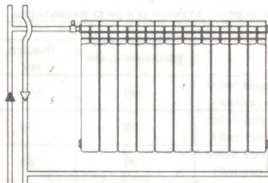
Боковая двухтрубная схема подключения
