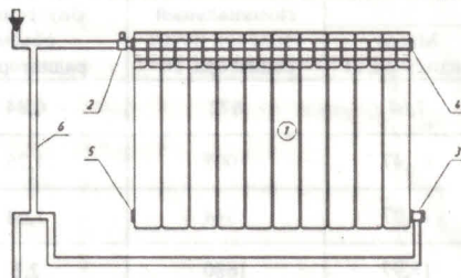
Боковая однотрубная схема подключения
