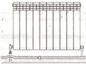
Нижняя двухтрубная схема подключения
